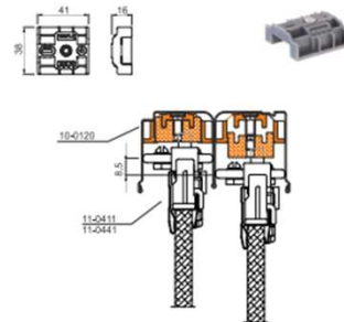
59-1690 Chwytyk domykacza Comfort Touch (40 szt.) Comfort Touch spring catch (40 pcs.) Doigt d'entraînement pour amortisseur Comfort Touch (40 pcs.)
